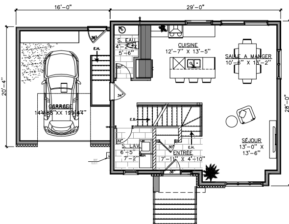
PLAN DE REZ-DE-CHAUSSÉE : 1 110 PI 2
