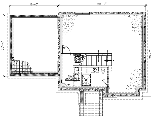
PLAN DE SOUS-SOL: 784 PI 2
