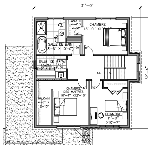
PLAN DE L'ÉTAGE: 923 P12
