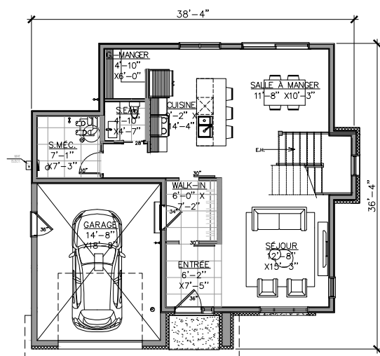
PLAN DE REZ-DE-CHAUSSÉE : 1 200 P12
