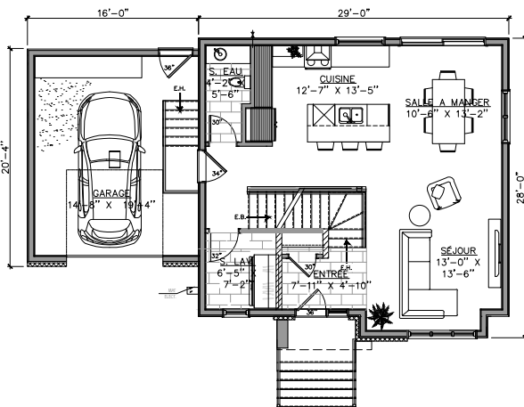
PLAN DE REZ-DE-CHAUSSÉE : 1104 PI2
