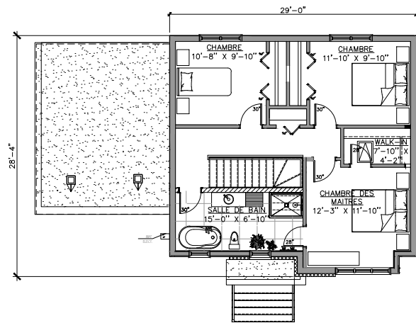
PLAN DE L'ÉTAGE: 779 PI2
