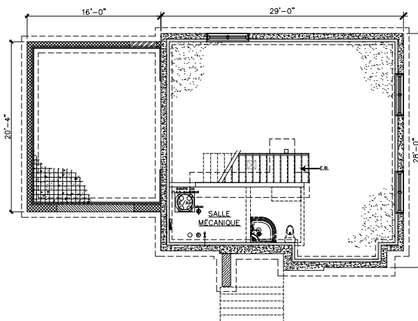
PLAN DE SOUS-SOL: 779 PI2
