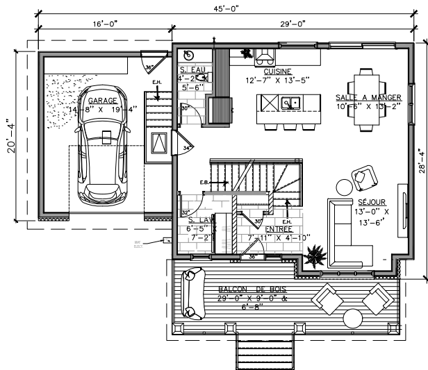
PLAN DE REZ-DE-CHAUSSÉE : 1110 PI 2
